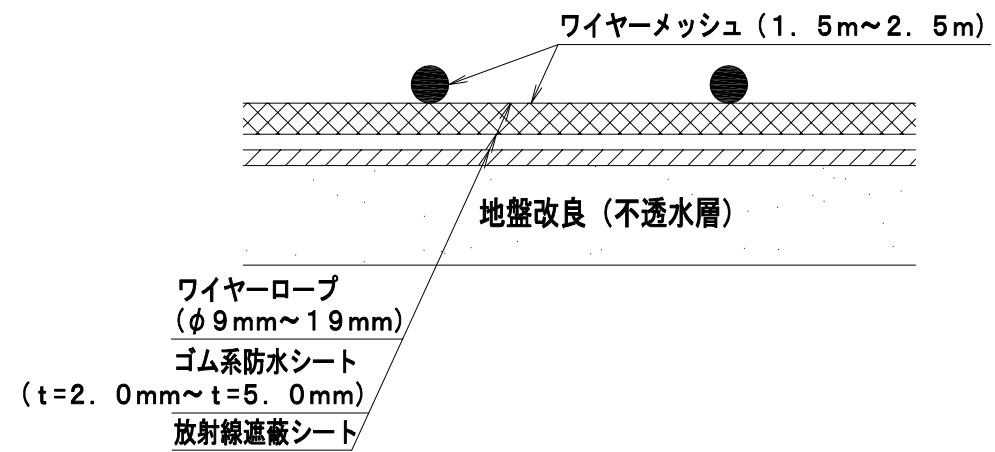
a 部 詳細
